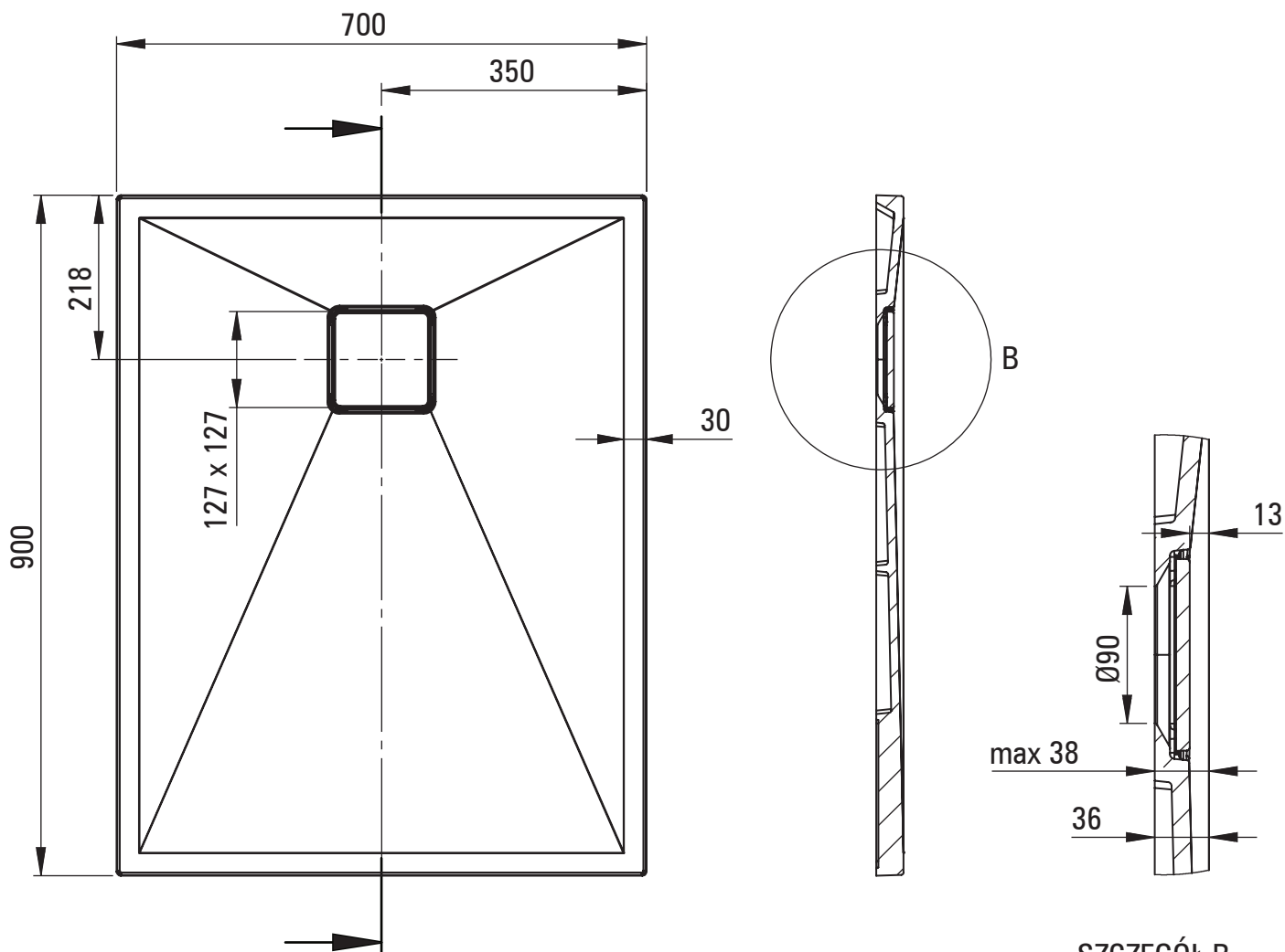
SZCZEGÓŁ B SKALA 1 : 5
