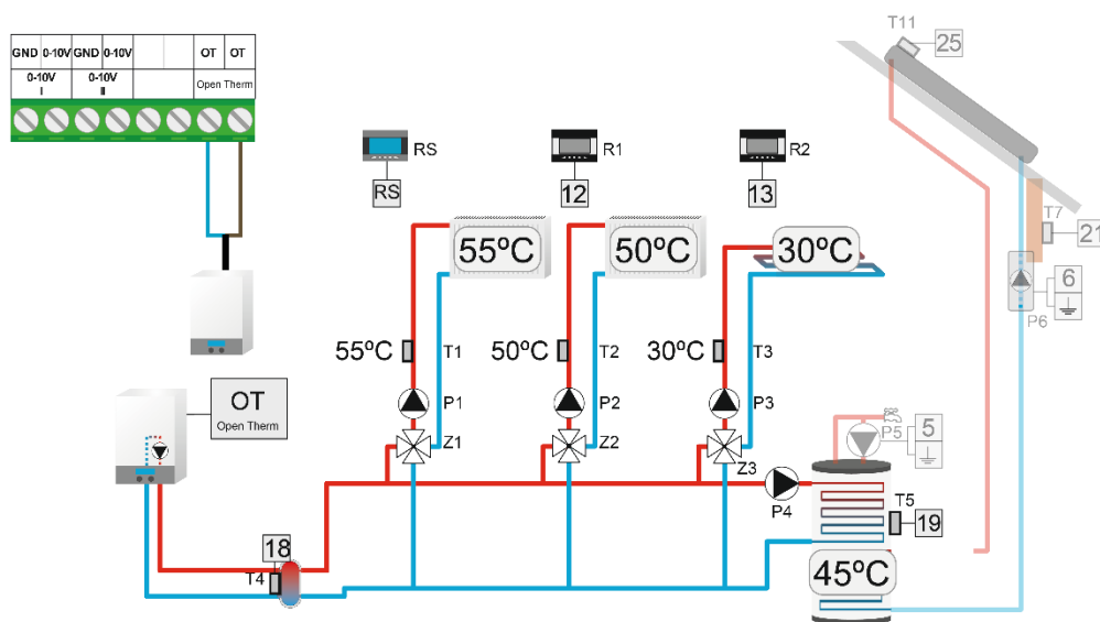
Przykład instalacji obsługiwanej za pomocą protokołu Open Therm.
