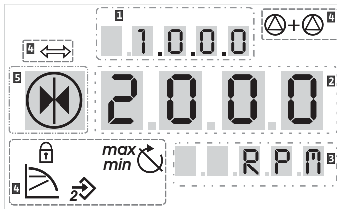
Rys. 30: Struktura wyświetlacza
