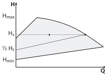
Kuva 11: Säätö \Delta p -v
