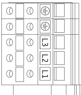
Kuva 26: Teholiittimet (verkkoliittimet)
