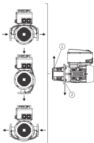
Kuva 18: Sallitut asennusasennot, vaakasuora moottoriakseli
