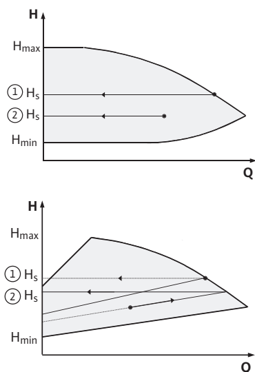
Fig. 43: Reglering \Delta p-c/\Delta p-v
