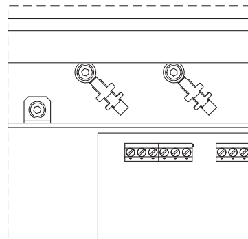
Fig. 24: Kabelavskärmning
