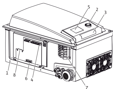
Kuva 9: Elektroniikkamoduuli
