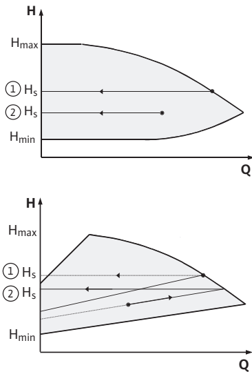
Kuva 43: Säätö \Delta p-c/\Delta p-v
