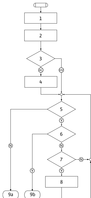
Fig. 54: Feltyp E, schema
