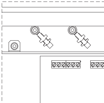
Rys. 24: Ekranowanie przewodu
