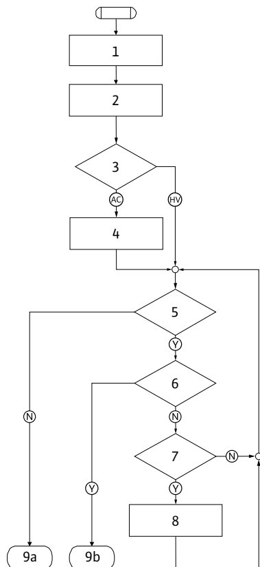
Fig. 53: Typ błędu E, schemat
