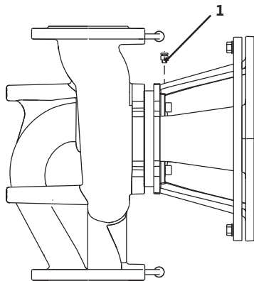
Fig. 40: Avluftningsventil
