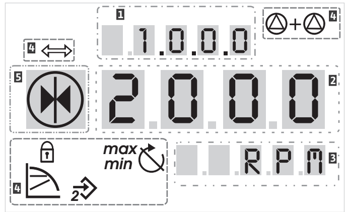
Fig. 29. Структура дисплея
