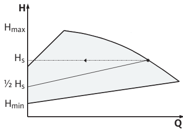
Fig. 11: Säättö \Delta p -v
