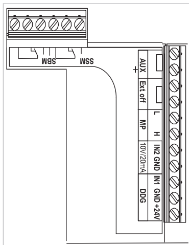
Fig. 24: Ohjauspäätteet
