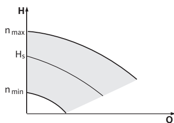
Fig. 43: Tryb sterowania
