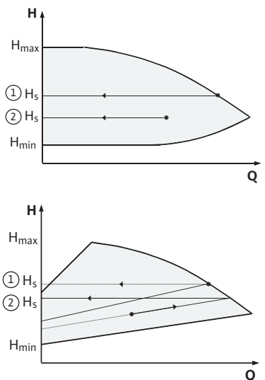
Fig. 42: Reglering \Delta p-c/\Delta p-v
