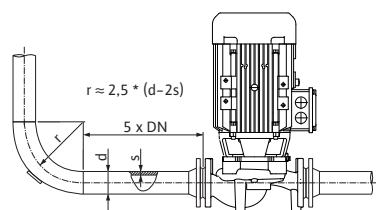
Fig. 21: Kevennysmatka ennen pumppua ja pumppun jälkeen
