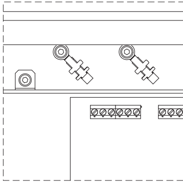
Fig. 23: Ekranowanie przewodu
