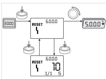
Fig. 44: Navigointi vikatapauksessa
